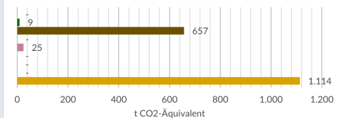
THG-Emissionen Basisjahr
