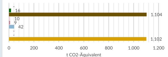
THG-Emissionen Basisjahr
