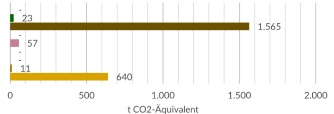
THG-Emissionen Basisjahr
